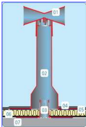
instalace komínku 1107P
