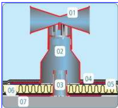
instalace komínku 1105P
