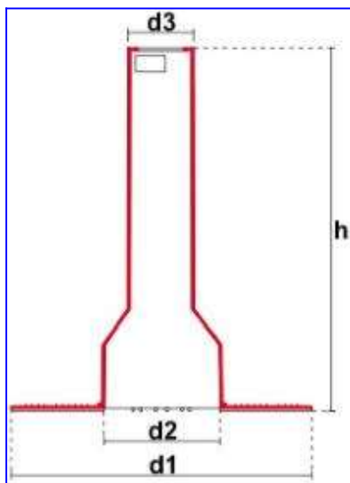
větrací komínek 1107P
