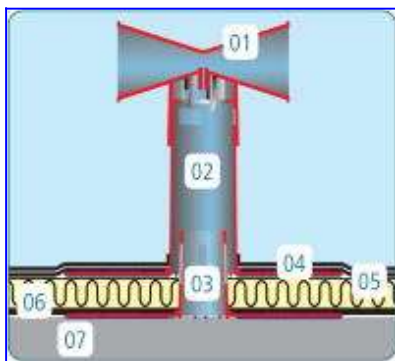
instalace komínku 1108P
