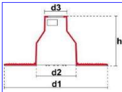
větrací komínek 1105P
