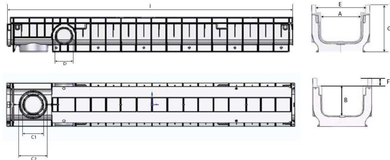
rozměry žlábků TAURUS
